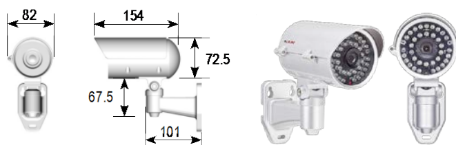
日夜兩用720P AHD紅外線攝影機
