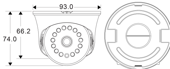
機身尺寸
