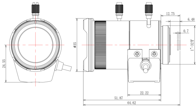
鏡頭尺寸圖 (mm)：
