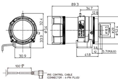
鏡頭尺寸圖 (mm) :
