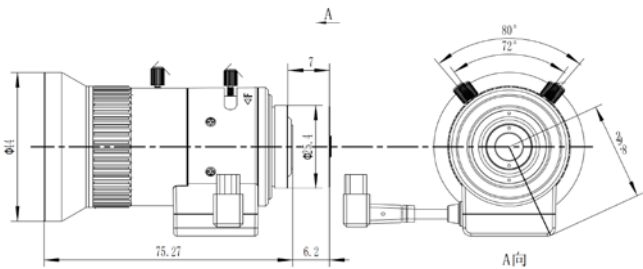
鏡頭尺寸圖（mm）：
