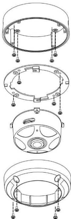
吸頂式結構圖 (吸頂式底座為選購品)
