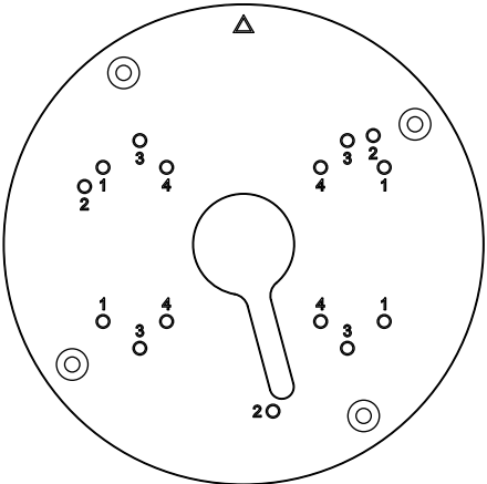
HOLE POSITION DIAGRAM 孔位圖
