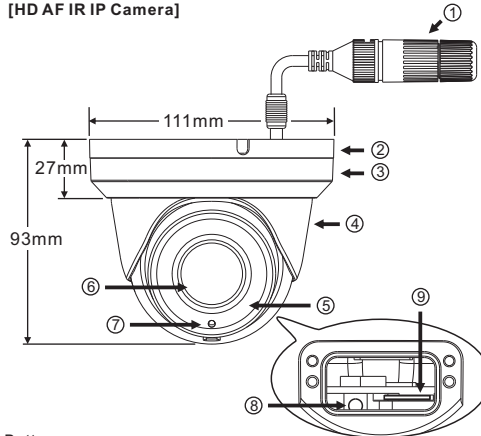
[HD AF IR IP Camera]
