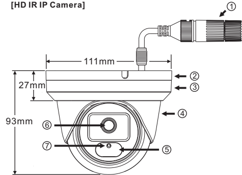
[HD IR IP Camera]
