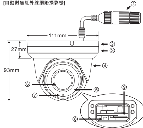
[自動對焦紅外線網路攝影機]
