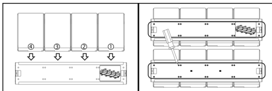
將硬碟鎖於硬碟支架上
