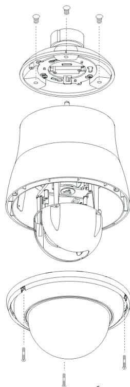
〔組裝示意圖〕
